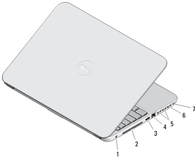
4. ábra. Hátnézet
